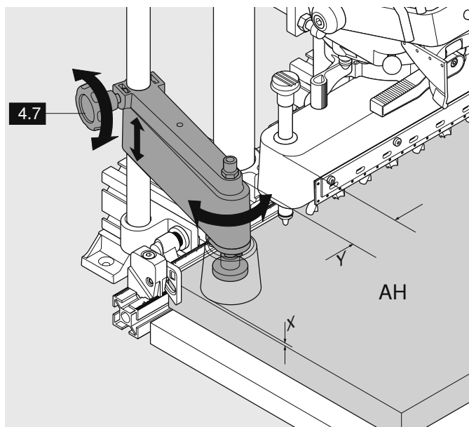
4.7 - Ajuste los prensapanes al grosor del material
