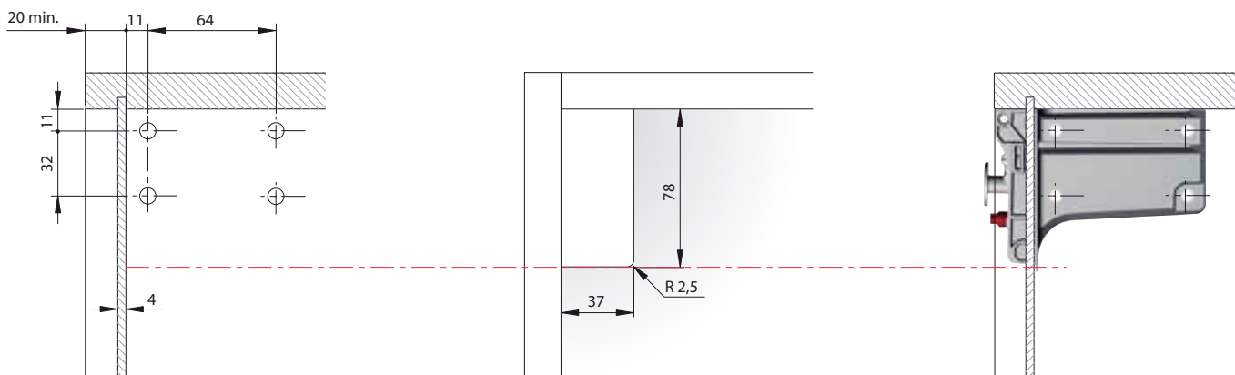
Perforación con panel trasero de 4 MM de espesor
