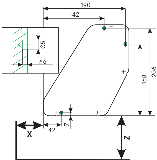
Esquema de taladros para lengüetas de posicionamiento
