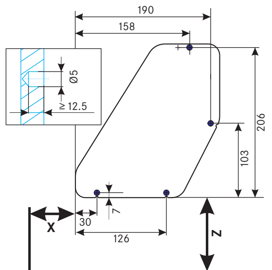
Esquema de taladros para tornillos euro
